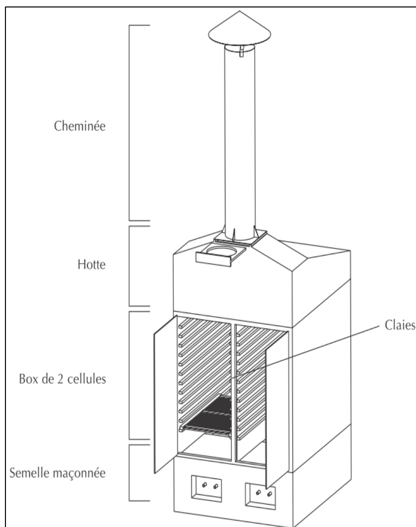
FIGURE 7.8. SÉCHOIR TRADITIONNEL À CONVECTION NATURELLE DITS "ATESTA" (RIVIER ET AL., 2009)
