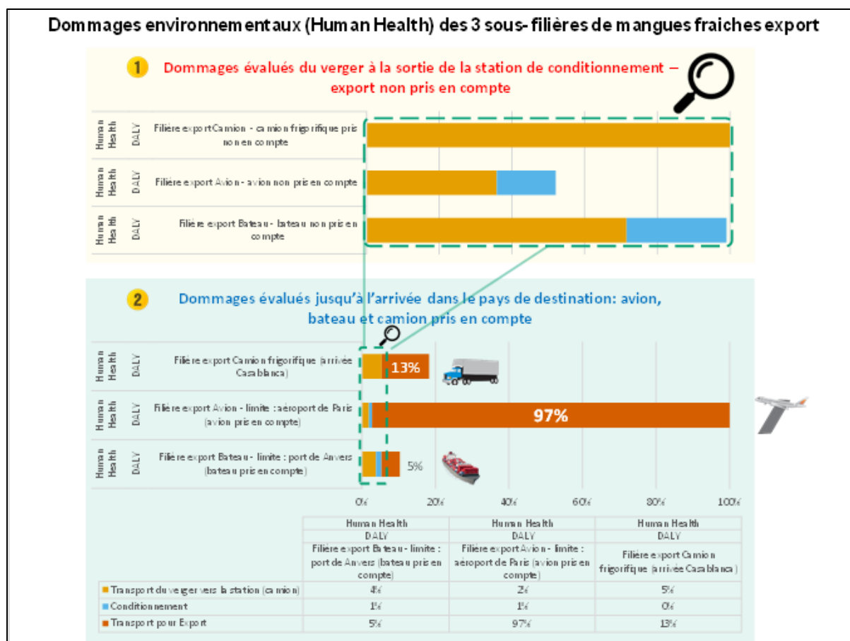
FIGURE 4.13 : DOMMAGES ENVIRONNEMENTAUX (HUMAN HEALTH) DES 3 SOUS-FILIÈRES DE MANGUES FRAÎCHES EXPORT, EXPRIMÉS DE DEUX FAÇONS : 1) AVEC LA LIMITE À LA STATION DE CONDITIONNEMENT ET 2) AVEC LA LIMITE AU PAYS DE DESTINATION.
