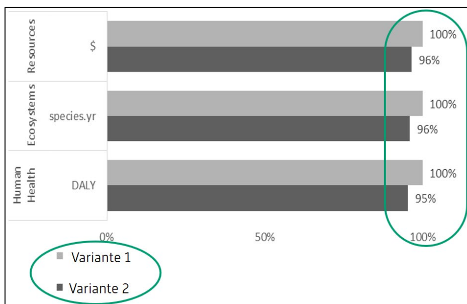
FIGURE 4.5 : REPRÉSENTATION DES RÉSULTATS D'UNE COMPARAISON DE VARIANTES DE SYSTÈMES (NON RÉALISABLE AVEC DES SYSTÈMES À UNITÉS FONCTIONNELLES DIFFÉRENTS)
