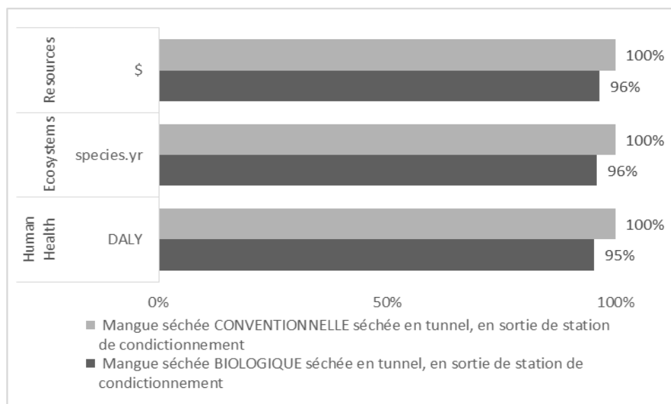
Figure 4.7 : Comparaison des dommages environnementaux de la mangue séchée biologique et conventionnelle avec le même mode de séchage
