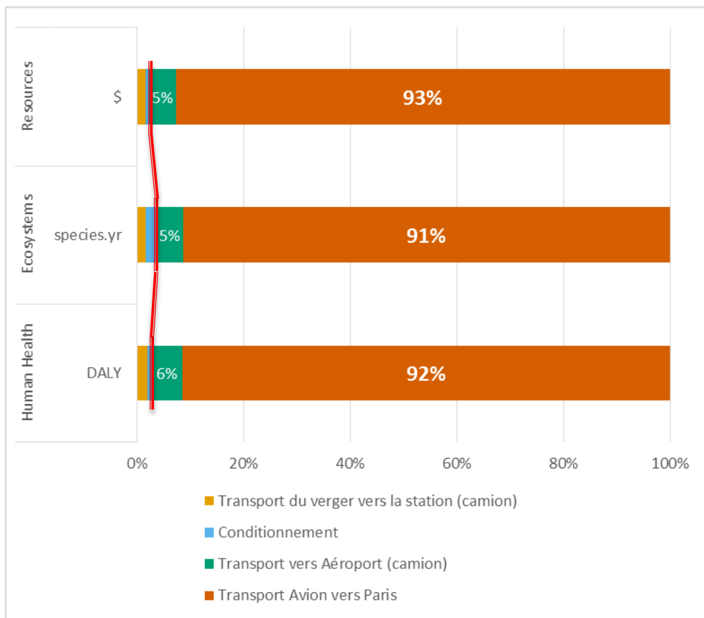
FIGURE 4.10 : ANALYSE DE CONTRIBUTION, AVEC PRISE EN COMPTE DE L'EXPORT AVION (ARRIVÉE À PARIS) - MANGUE FRAICHE EXPORTÉE
