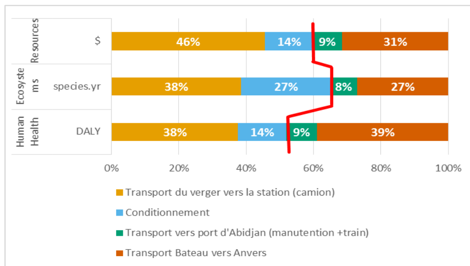
FIGURE 4.11 : ANALYSE DE CONTRIBUTION, AVEC PRISE EN COMPTE DE L'EXPORT EN TRAIN VERS ABIDJAN + BATEAU (ARRIVÉE À ANVERS) - MANGUE FRAICHE EXPORTÉE
