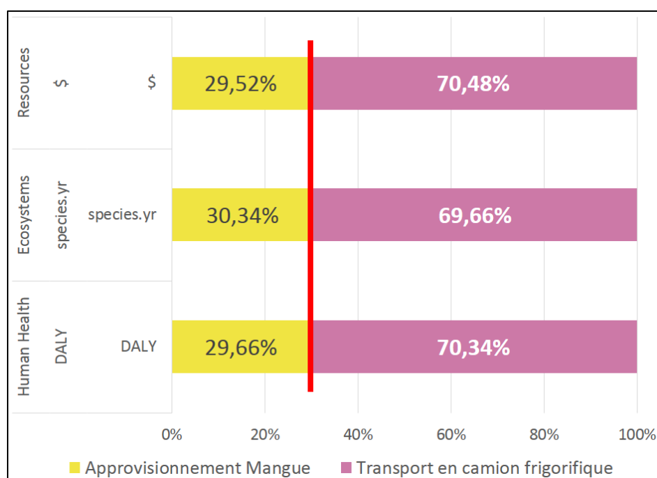
FIGURE 4.12 : ANALYSE DE CONTRIBUTION POUR 1 KG DE MANGUE FRAICHE EXPORTÉE VERS LE MAROC PAR CAMION FRIGORIFIQUE (ARRIVÉE : CASABLANCA)
