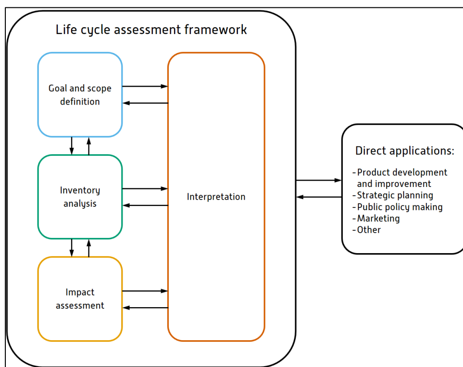
FIGURE 4.1 : LES 4 ÉTAPES CLASSIQUES DE LA MÉTHODE ACV
