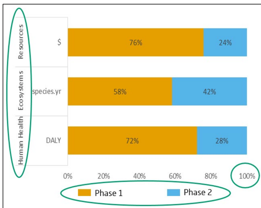
FIGURE 4.4 : REPRÉSENTATION DES RÉSULTATS SOUS FORME D'UNE ANALYSE DE CONTRIBUTION DES PRINCIPALES PHASES D'UN PROCESS
