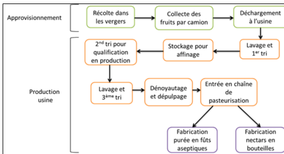
FIGURE 1.11. FONCTIONNEMENT DE L'UNITÉ DE FABRICATION DE PURÉE ET DE NECTARS (POMMIER, 2014)
