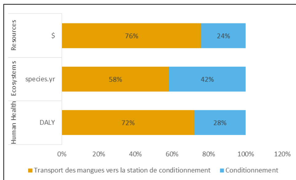
FIGURE 4.6 : ANALYSE DE CONTRIBUTION DES PRINCIPALES PHASES POUR LA MANGUE FRAICHE EXPORT (LIMITES = SORTIE DE STATION DE CONDITIONNEMENT)
