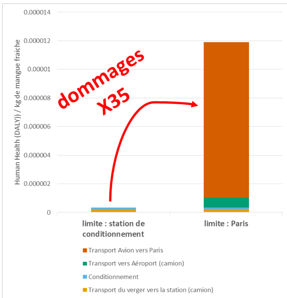
FIGURE 4.9 : MISE EN ÉVIDENCE DE L'EFFET DE LA LIMITE SUR LE SYSTÈME CHOISI, ILLUSTRÉE SUR LA SANTÉ HUMAINE, POUR 1 KG DE MANGUE FRAICHE EXPORTÉE PAR AVION VERS L'EUROPE
