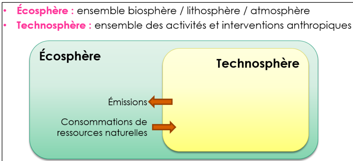
FIGURE 4.3 : FORMALISME CLASSIQUE DE QUANTIFICATION DES FLUX ÉLÉMENTAIRES EN ACV
